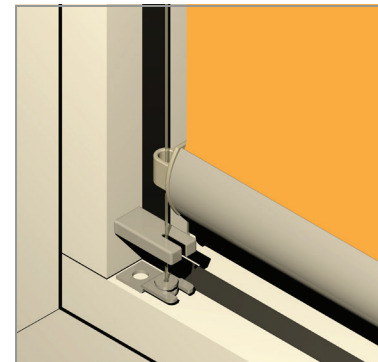
Staffa piatta + Copristaffa (fissaggio a soffitto)
