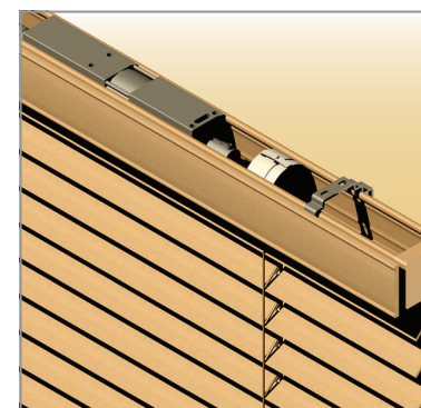
Versione con Motore (misure realizzabili max. 5 mq.)
