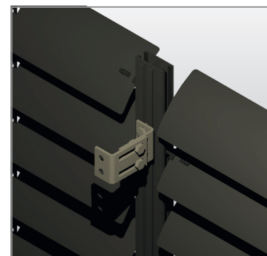
Mensola per fissaggio guida doppia
