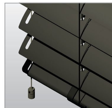
Guida in acciaio rivestito Ø 2,5 mm con Morsettone (a richiesta)
