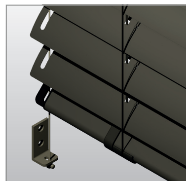
Guida in acciaio rivestito Ø 2,5 mm con Staffa a "L" Inox (a richiesta)
