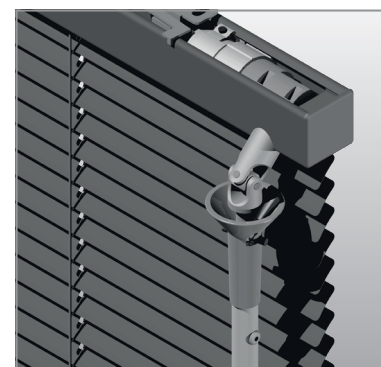
Innesto per asta sganciabile (su richiesta)
